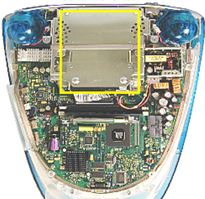
CD-ROM/DVD ROM
