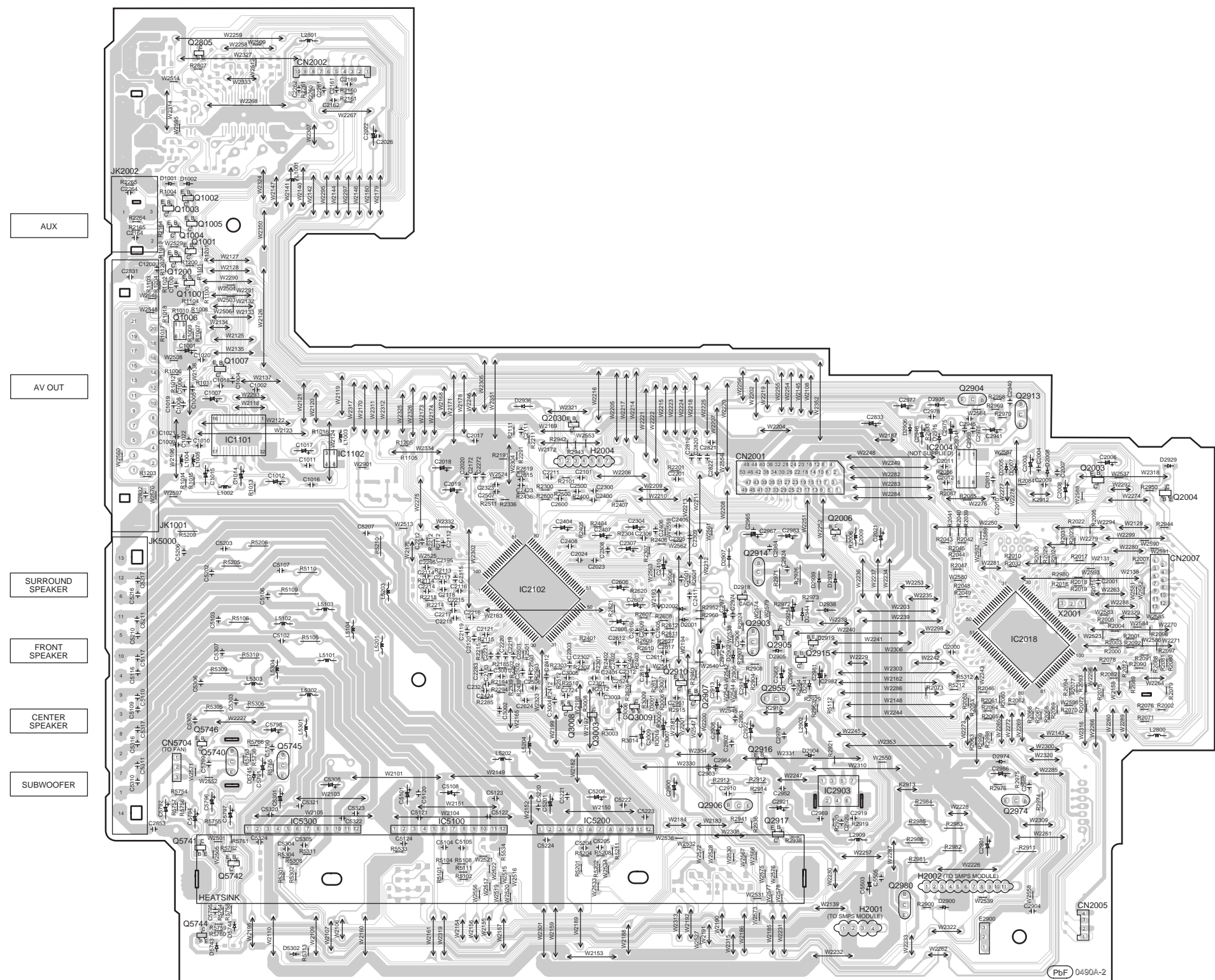
B MAIN P.C.B. (REPX0531A)
